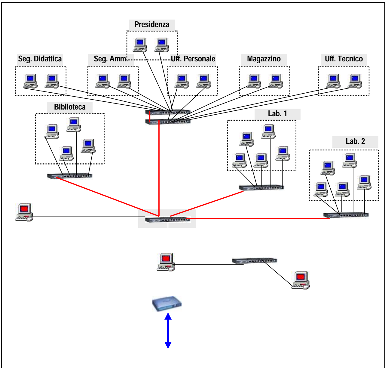
Schema cablaggio strutturato
