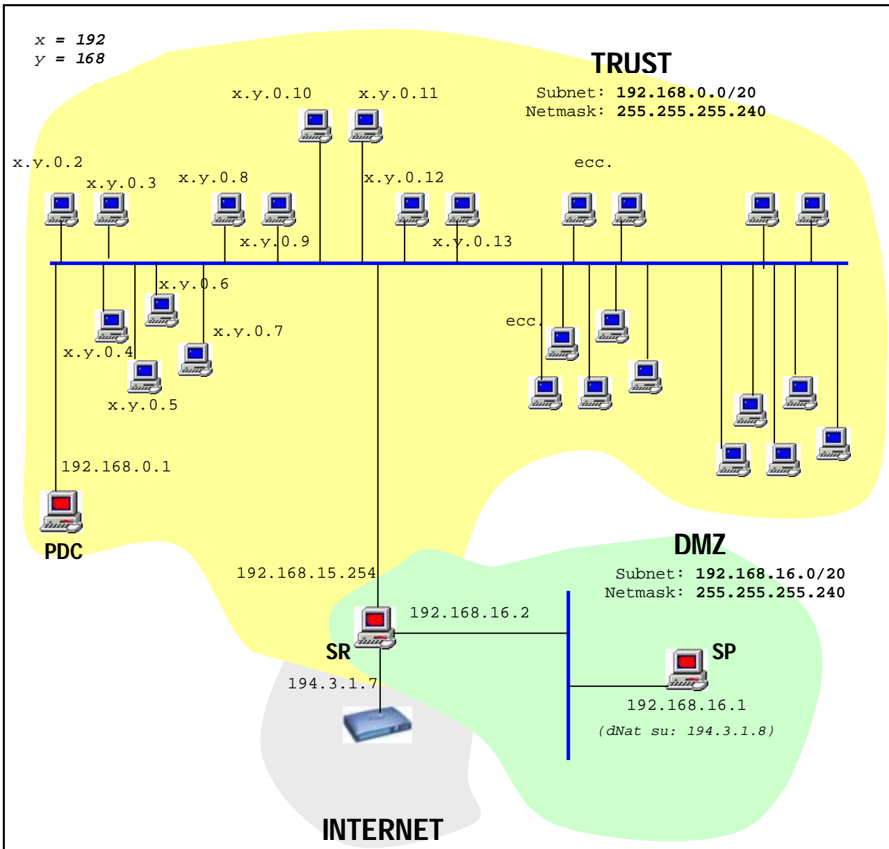
Schema topologia e indirizzamento
