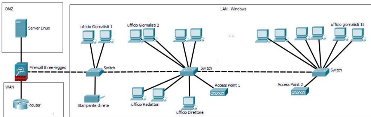
Schema dell'infrastruttura di rete
